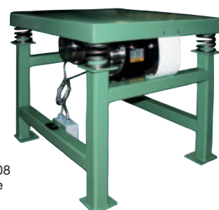
VT 7/8 mit 2 NEG 50770 elektrisch
